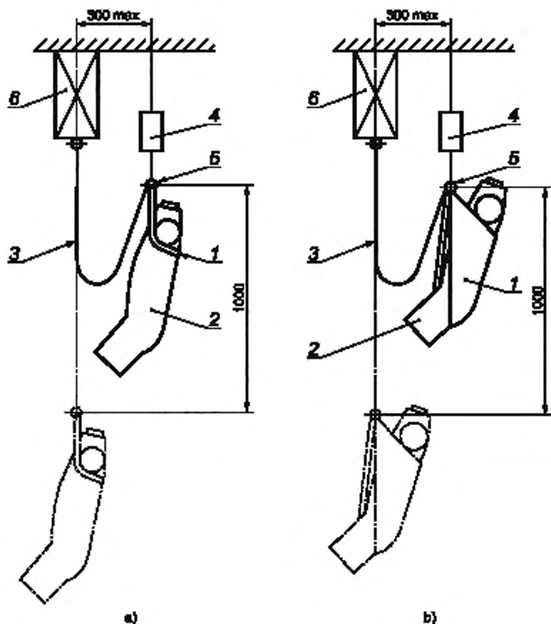
а) — класс А; б) — класс В; 1 — спасательная петля; 2 — манекен корпуса человека; 3 — испытательная стропы; 4 — устройство быстрого расцепления; 5 — элемент крепления; 6 — испытательное оборудование
