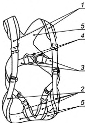
1 — основные наплечные ляжки; 2 — основные набедренные ляжки; 3 — основные ляжки; 4 — место подсоединения (включающее два элемента крепления), 5 — мягкий протектор
