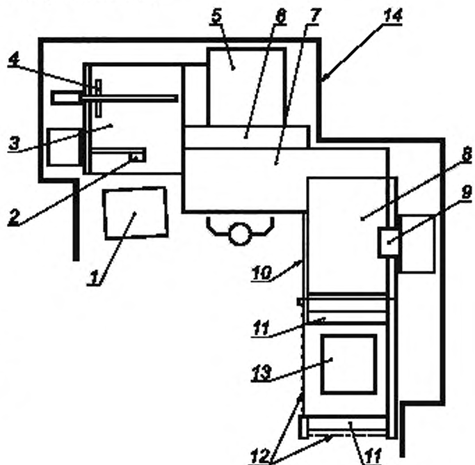
1 — бумажный сталець; 2 — щипцовый захват; 3 — загрузочный стол; 4 — толкатель; 5 — задний стол; 6 — машина резальная; 7 — передний стол; 8 — разгрузочный стол; 9 — прижим; 10 — ограждение; 11 — приемный упор; 12 — ЭЧПУ; 13 — поддон; 14 — ограждение
