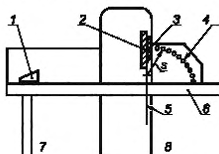
Рисунок 2 — ЭЧПУ машины резальной одноножевой
