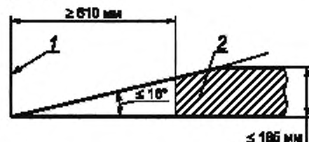
Рисунок 4 — Расположение переднего светового луча ЭЧПУ
