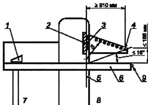
Рисунок 3 — ЭЧПУ с двуручным управляющим устройством
