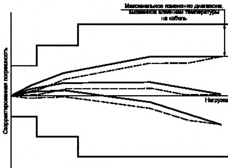
Рисунок 12 — Изменение диапазона из-за влияния температуры на кабель
