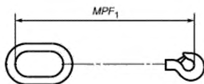
а) Стропальная цепь из одного жгута
