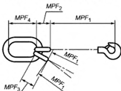
в) Стропальная цепь из трех жгутов
