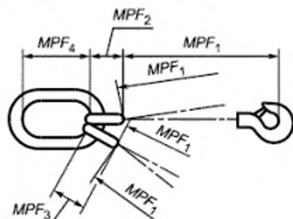
г) Стропальная цепь из четырех жгутов
