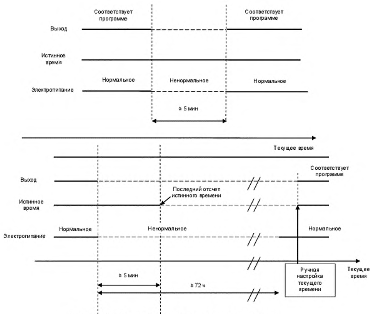
Рисунок 7 – Временная диаграмма защиты данных
