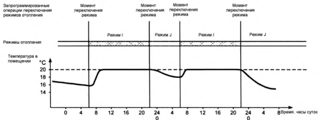
Рисунок 1 – Пример соотношения между периодами пребывания людей, режимами отопления и температурой в помещении.
