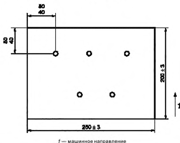
Рисунок 1 — Расположение точек на испытываемом образце для измерения средней толщины образцов
