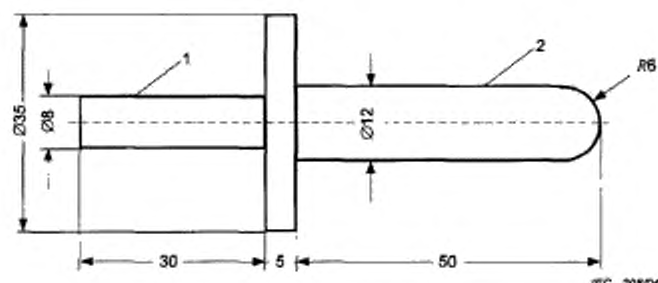
Рисунок 104 — Минимальные размеры (в мм) защитного устройства задней рукоятки
