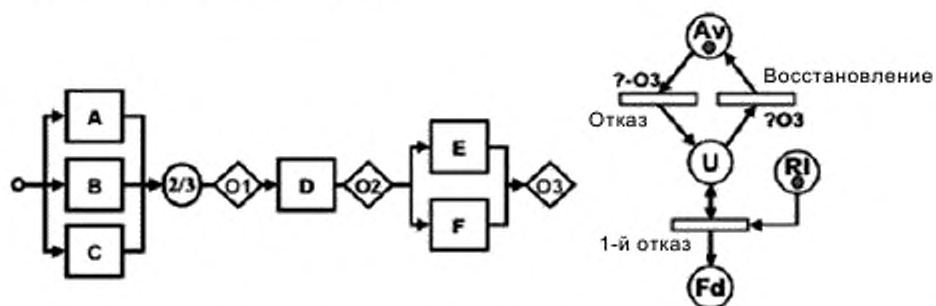
Рисунок В.35 – Использование блок-схемы надежности для построения сети Петри и вспомогательной сети Петри для вычислений PFd и PFH
