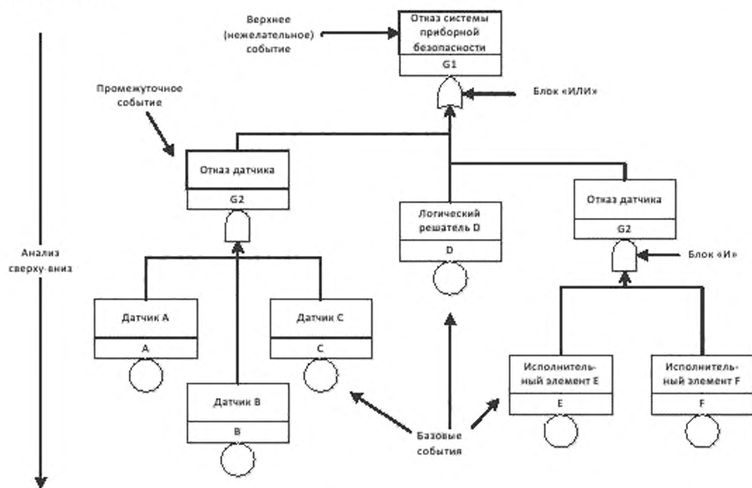
Рисунок В.17 – Простое дерево отказов, эквивалентное блок-схеме, представленной на рис. В.1
