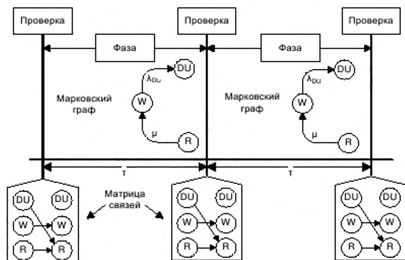
Рисунок В.24 – Принцип марковского многофазного моделирования
