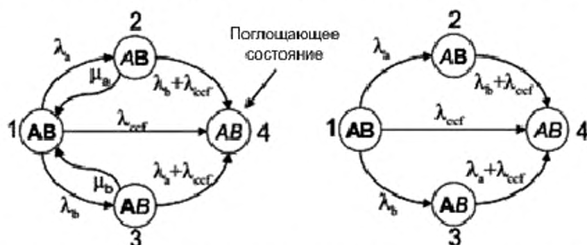
Рисунок В.31 – Марковский граф «надежности» с поглощающим состоянием
