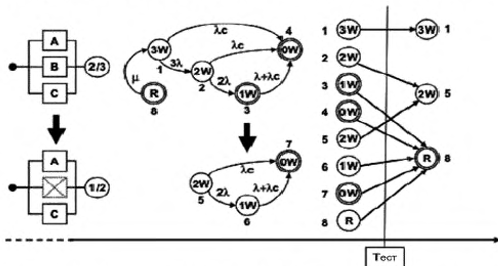
Рисунок В.30 – Изменение логики (с 2oo3 на 1oo2) вместо ремонта первого отказа
