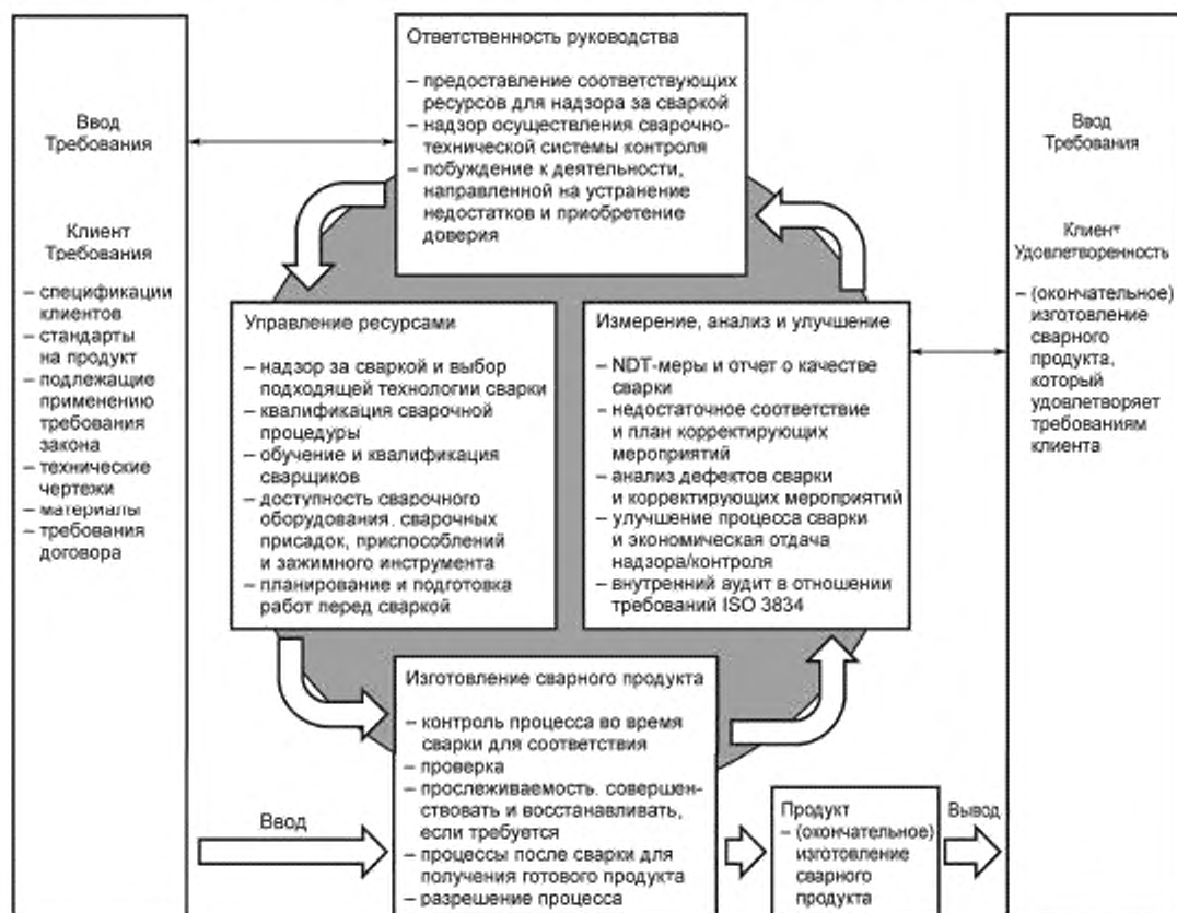
Рисунок 1 — Модель системы управления сварочным производством
