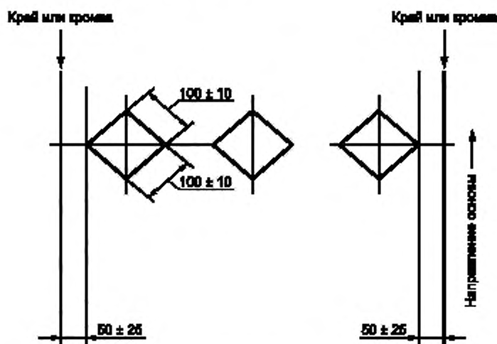
Рисунок 8 — Места вырезки образцов при определении содержания смолы
