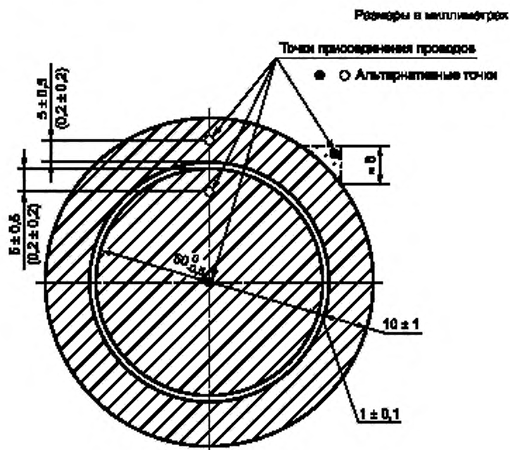
Рисунок 27 — Рисунок электродов круглой формы
