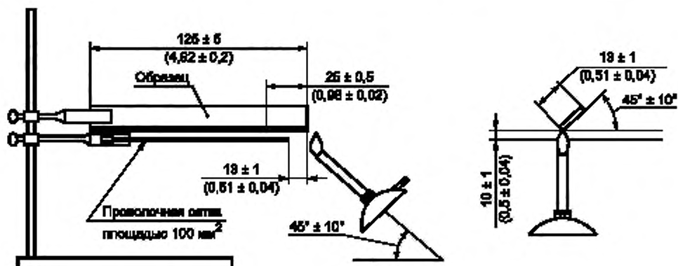
Рисунок 4 — Стенд для испытаний
