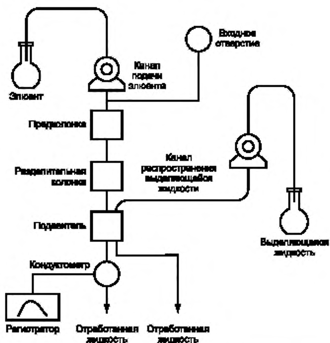
Рисунок 10 — Структура хроматографа с системой ионного обмена
