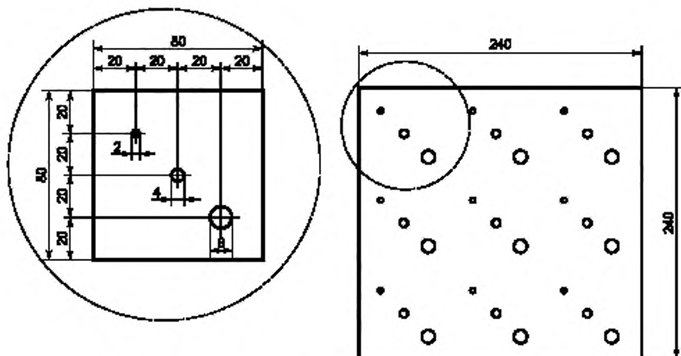
Рисунок 19 — Перфорированный тестовый рисунок для метода выдавливания
