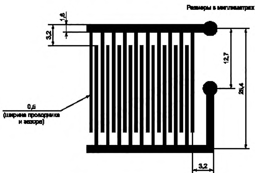
Рисунок 28 — Рисунок электродов гребенчатой формы
