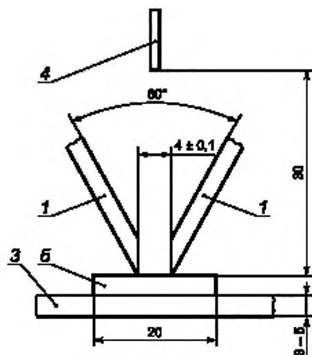
1 — электрод платиновый; 3 — опора (стеклянная); 4 — источник капель; 5 — образец
