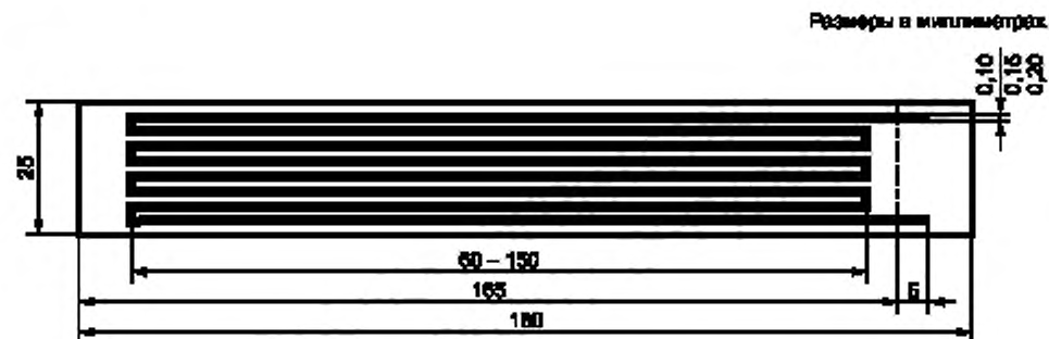
Рисунок 14 — Рисунок образца для испытаний
