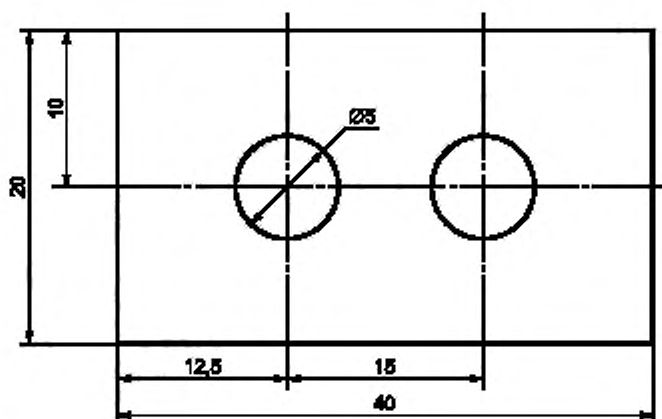
Рисунок 35 — Образец для проведения испытаний на сопротивление изоляции
