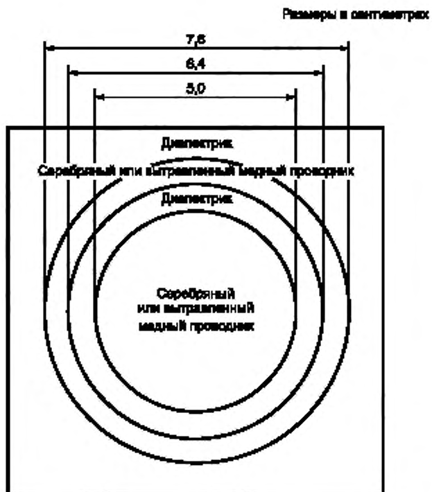
Рисунок 22б — Тестовый рисунок для определения объемного и поверхностного сопротивлений (сторона 1)
