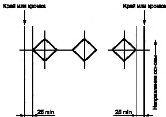
Рисунок 2 — Места вырезки образцов
