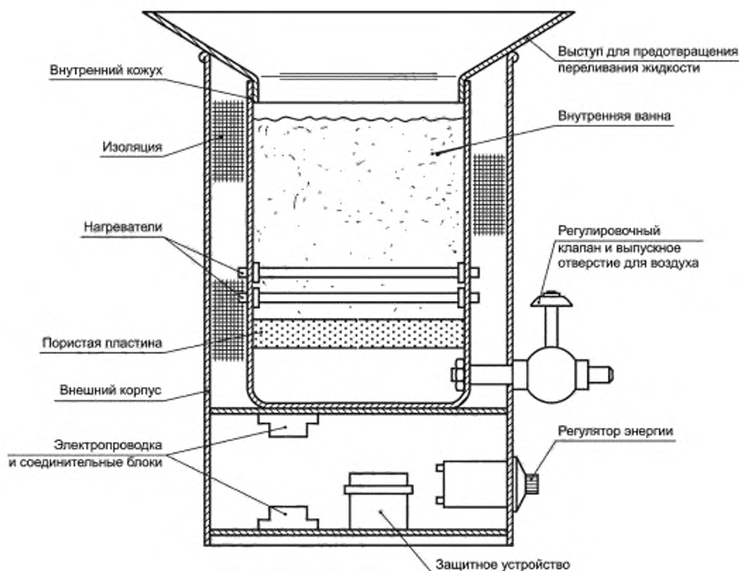
Рисунок 3 — Флюидизированная песочная баня. Принципы работы
