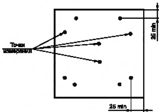
Рисунок 1 — Точки измерения толщины
