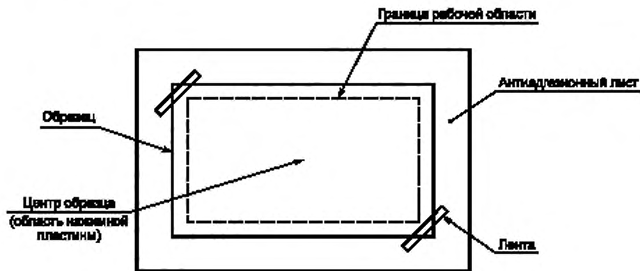
Рисунок 16 — Схема расположения образца перед прессованием
