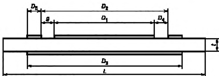
Рисунок 22а — Размеры тестового рисунка (см. таблицу 6)
