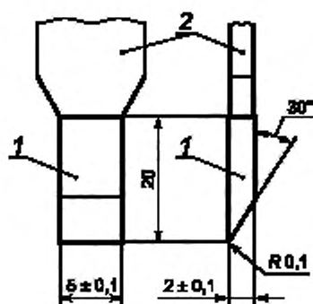
1 — электрод платиновый; 2 — удлинитель медный
