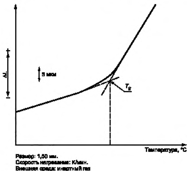
Рисунок 13 — Термомеханический анализ (в режиме расширения)
