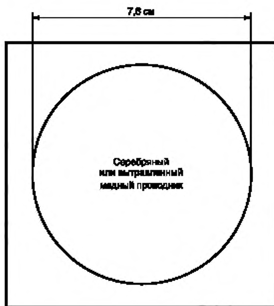
Рисунок 22с — Тестовый рисунок для определения объемного и поверхностного сопротивлений (сторона 2)
