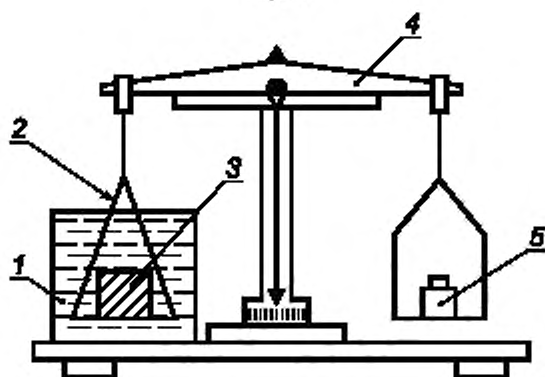
1 — сосуд с водой; 2 — подвес для образца; 3 — образец; 4 — весы; 5 — разновес
