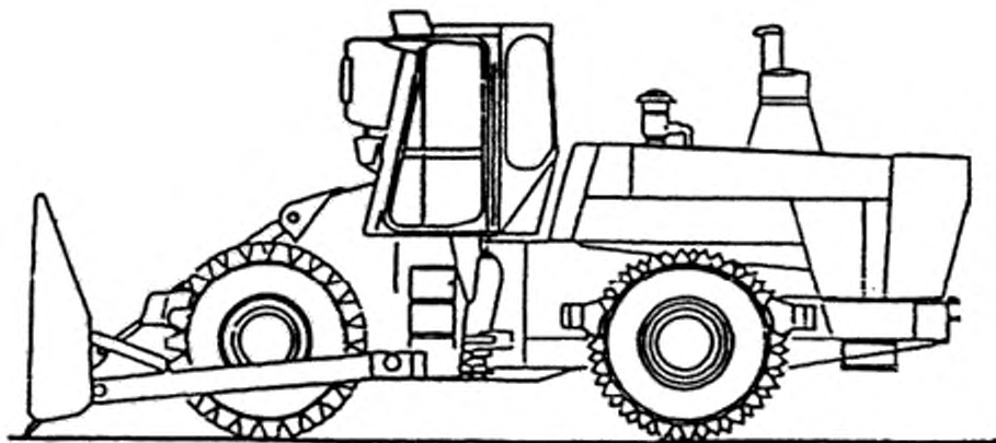
Рисунок В.2 – Уплотняющая машина с бульдозерным оборудованием
