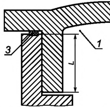
Рисунок 13 — Иллюстрация требований к прокладкам (пример 4)
