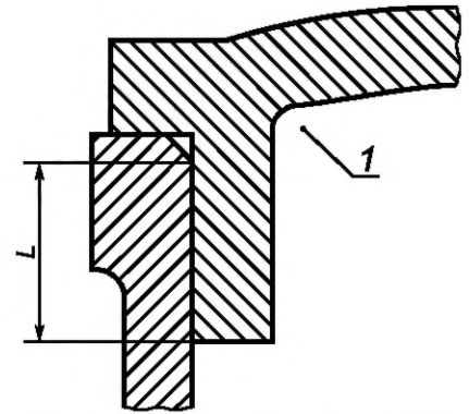
Рисунок 2b — Только Цилиндрическая часть
