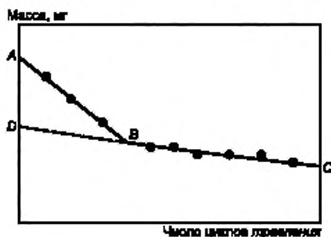
Рисунок 1 — График зависимости изменения массы прокорродированного образца после повторяющихся циклов удаления продуктов коррозии (травления)
