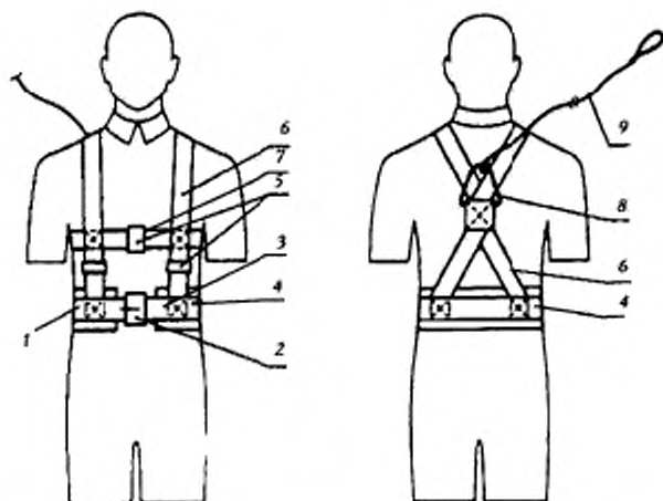
Рисунок 3 — Лямочный пояс, тип В (Ba)
