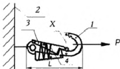
1 — основной крюк карабина; 2 — неподвижная опора; 3 — внутренняя рукоятка карабина; 4 — проволока диаметром 1—1,5 мм для закрепления рукоятки в указанном положении; P — растягивающее усилие ( 500 \pm 1 ) кгс; X — расстояние между наружной поверхностью носка крюка карабина и наружной поверхностью тыльной стороны крюка карабина; L — длина карабина, измеренная по оси приложения нагрузки
