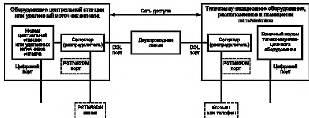
Рисунок А.1 — Типичная конфигурация xDSL системы
