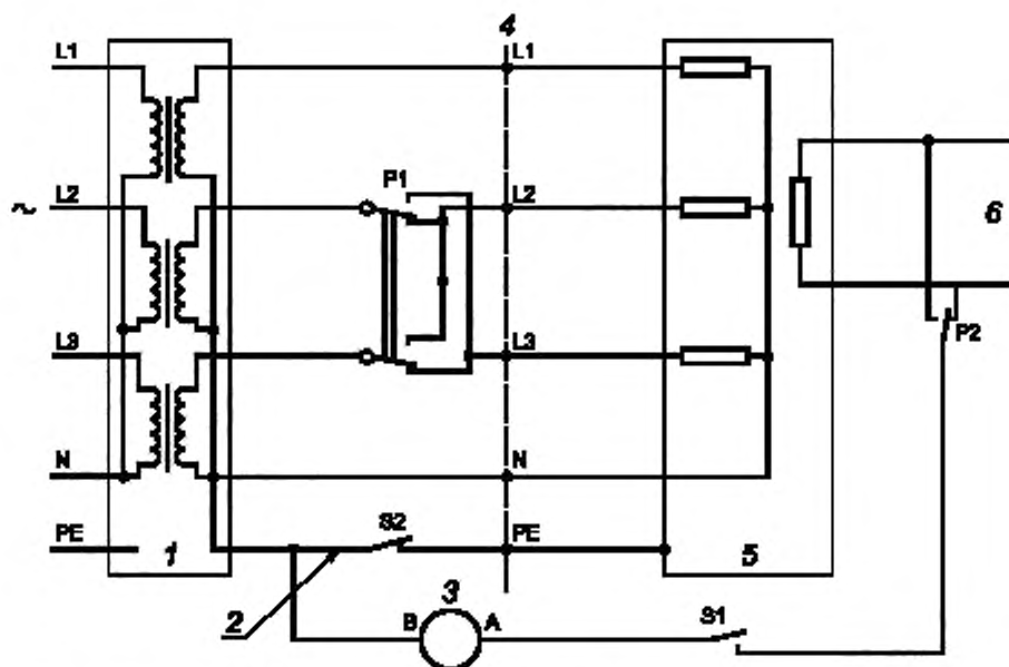
1 — изолирующий трансформатор (для измерений); 2 — провод заземления; 3 — измерительная щель; 4 — точка подключения к сети электропитания переменного тока; 5 — ИО; 6 — соединение с телекоммуникационной сетью (не подключено)
