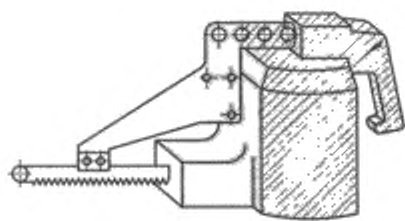
Рисунок 15 – Шаговая пила с полотном возвратно-поступательного действия
