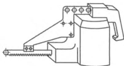
Рисунок 3 – Шаговая пила с полотном (возвратно-поступательного действия)
