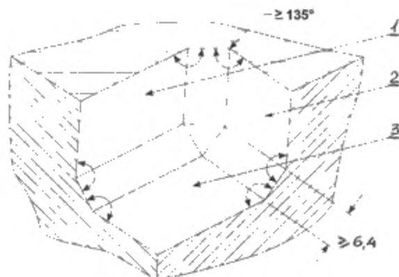
Рисунок В.4 – Соединение поверхностей в пищевой зоне
