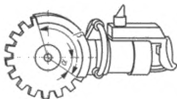
Рисунок 10 – Неподвижное защитное ограждение циркулярной пилы
