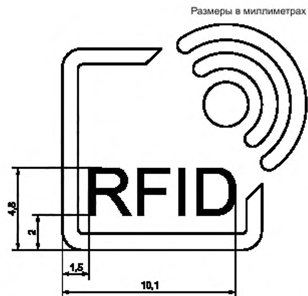
Рисунок В.2 — Универсальная эмблема радиочастотной идентификации
