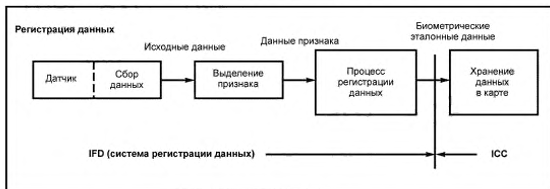
Рисунок А.1 — Общая схема процесса регистрации данных
