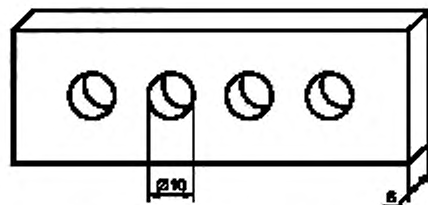
Рисунок 2 — Форма для образцов при испытании на текучесть
