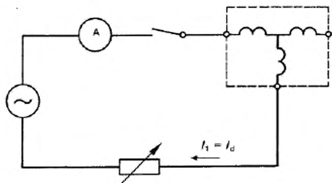
Рисунок 4В — Схема испытаний времени срабатывания
