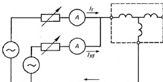
Рисунок 4С — Схема испытаний устойчивости к гармоническим составляющим
