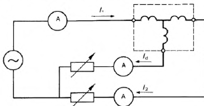
Рисунок 4А — Схема испытаний характеристик
