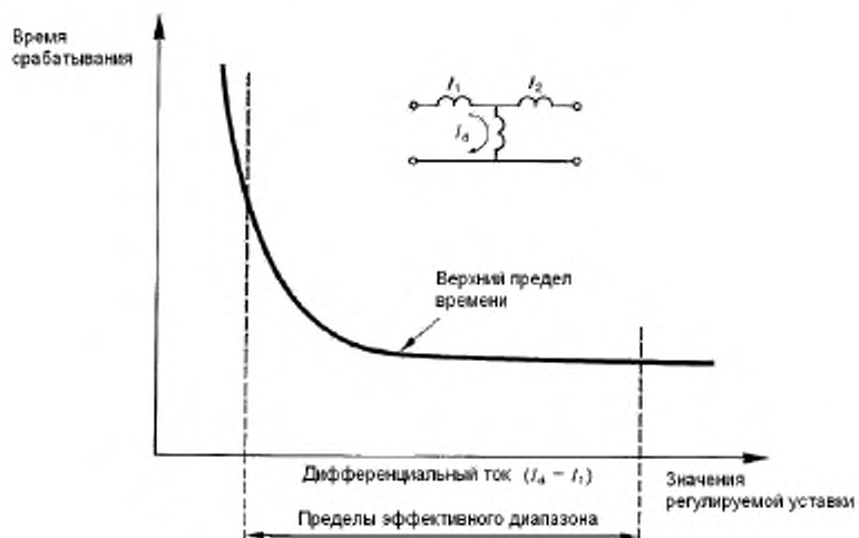
Рисунок 2 — Характеристика времени срабатывания в заданных условиях
