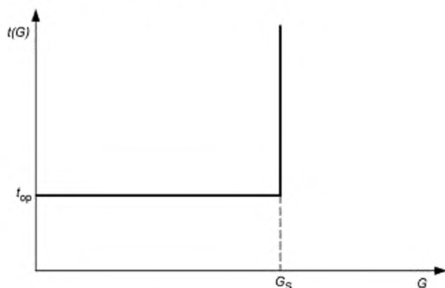
Рисунок 3 — Независимая характеристика времени реле минимального тока
