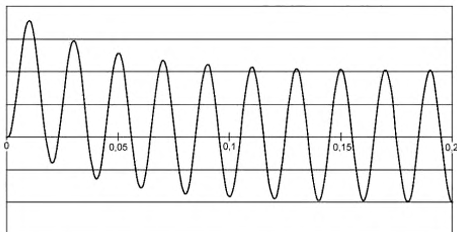
Рисунок 11 — Типичная испытательная оциллограмма кратковременных всплесков воздействия
