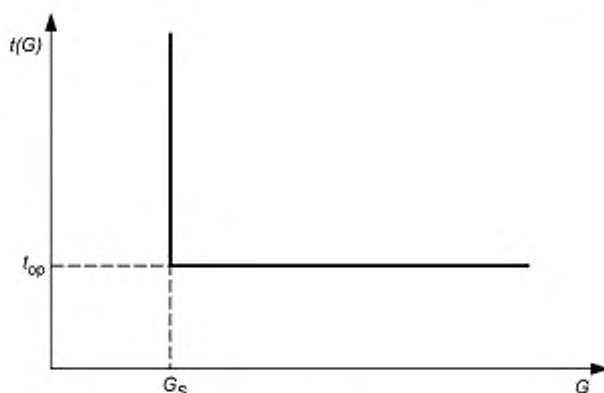
Рисунок 2 — Независимая характеристика времени реле сверхтока
