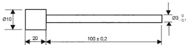
Рисунок 101 — Испытательный прут для скрытой блокировки
