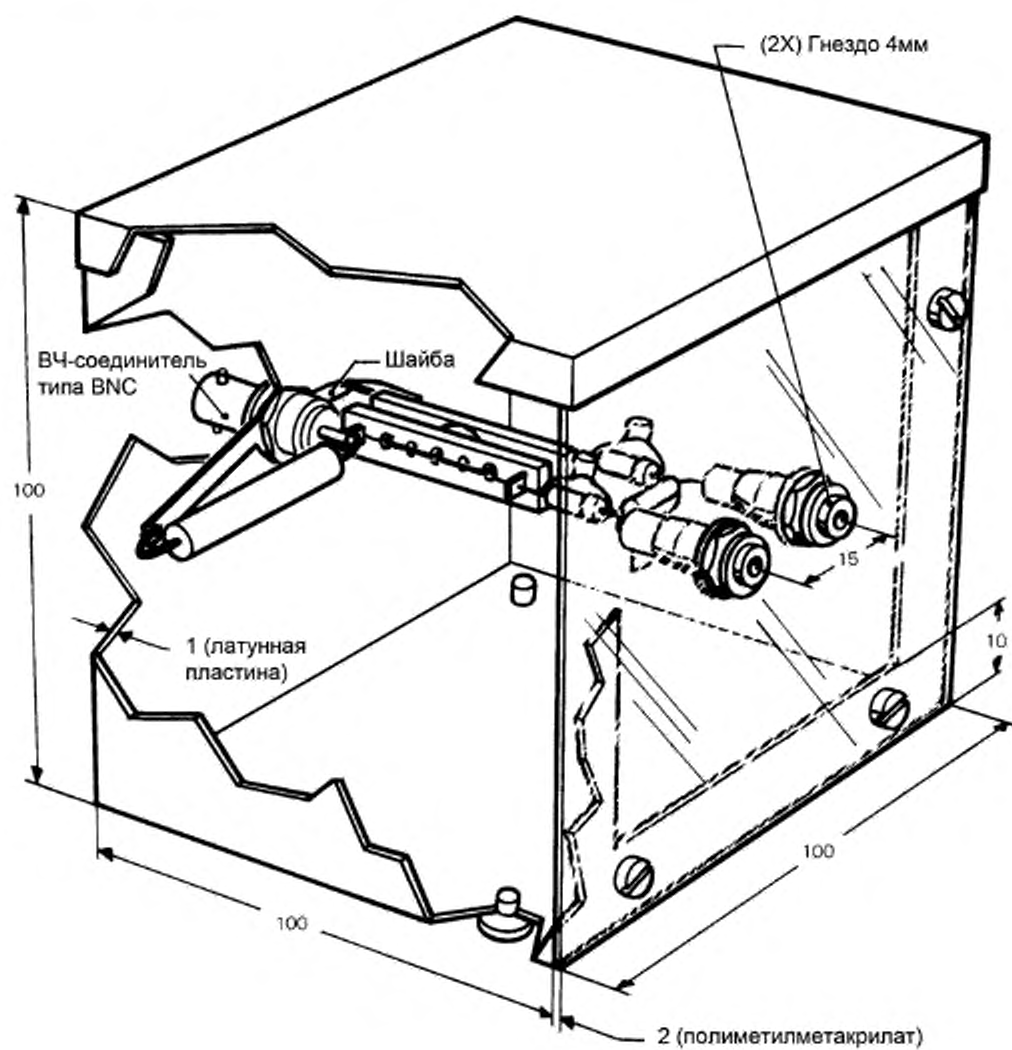
Рисунок А.2d – Конструкция трансформатора
