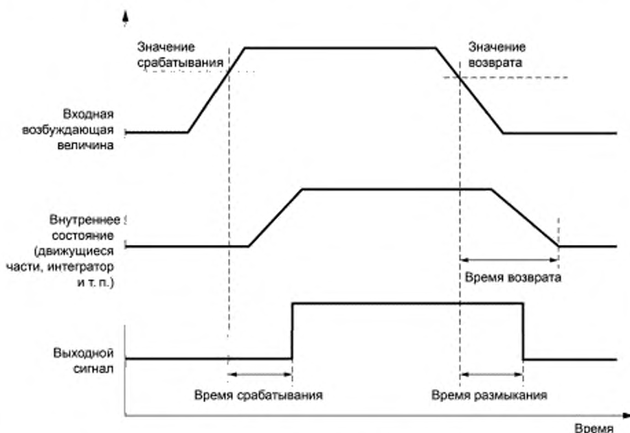
Рисунок 1 — Пояснительная диаграмма к терминам: время срабатывания, время размыкания и время возврата
