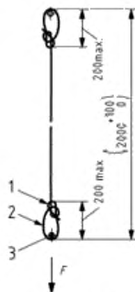
Рисунок 6 – Испытательная стропы для проверки прочности динамической нагрузкой
