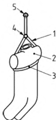
1 – спасательная петля, 2 – манекен корпуса человека, 3 – основная лямка; 4 – элемент подгоноки, 5 – элемент крепления
