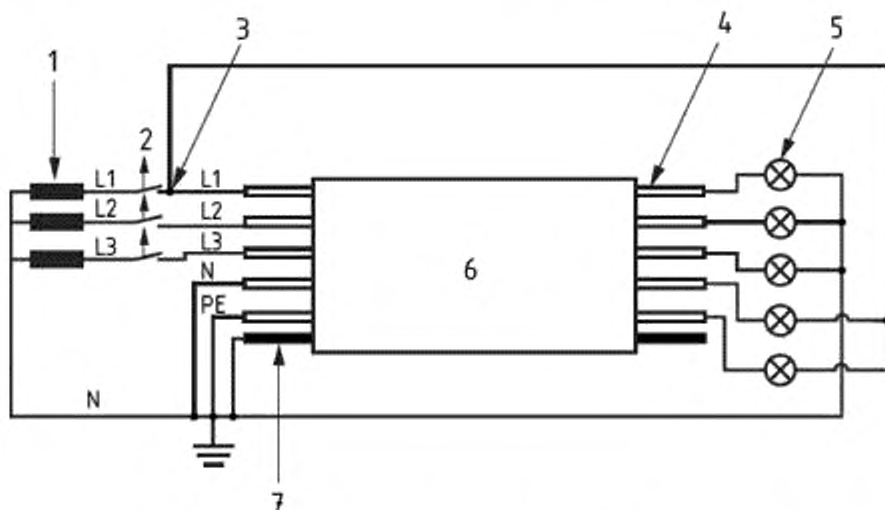
1 — трансформатор; 2 — плавкий предохранитель (2 А); 3 — фазы L1, L2 или L3; 4 — испытываемая жила или группа жил; 5 — нагрузочный индикаторный прибор; 6 — образец; 7 — металлический экран (при наличии); L1, L2, L3 — фазные жилы (L2, L3 при наличии); N — нейтральная жила (при наличии); PE — защитная жила (при наличии)
