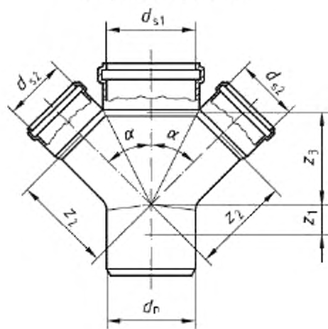
а) Крестовина
