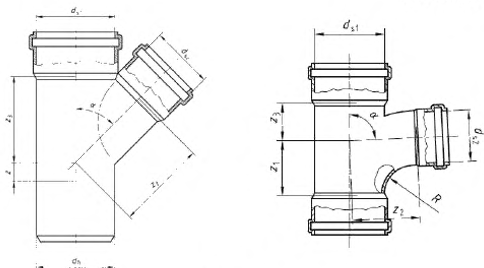
а) Тройник
