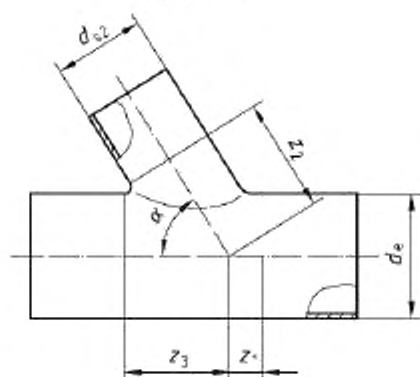
б) Тройник сварной Рисунок 6 – Тройники
