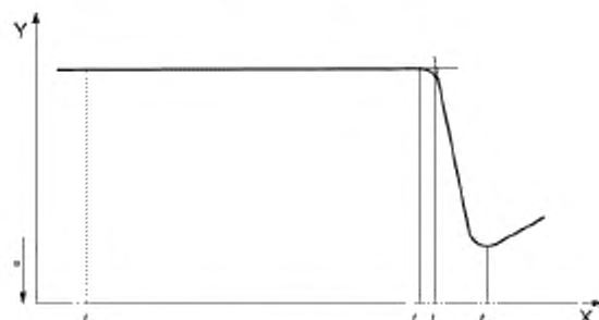
X – время; Y – тепловой поток; a – максимум экзотермы; t_1 – переключение на кислород или воздух (время ноль); t_2 – начало окисления; t_3 – точка определенная методом касательной; t_4 – максимум окисления
