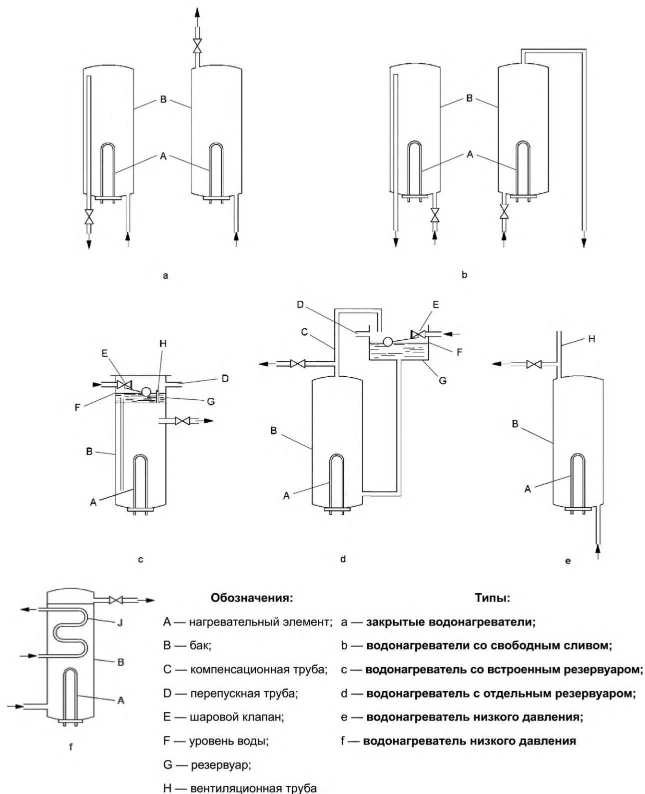
Рисунок 101 — Примеры типов аккумуляционных водонагревателей
