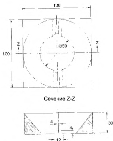
Рисунок 113б – Фрагмент В – Верхняя часть маски
