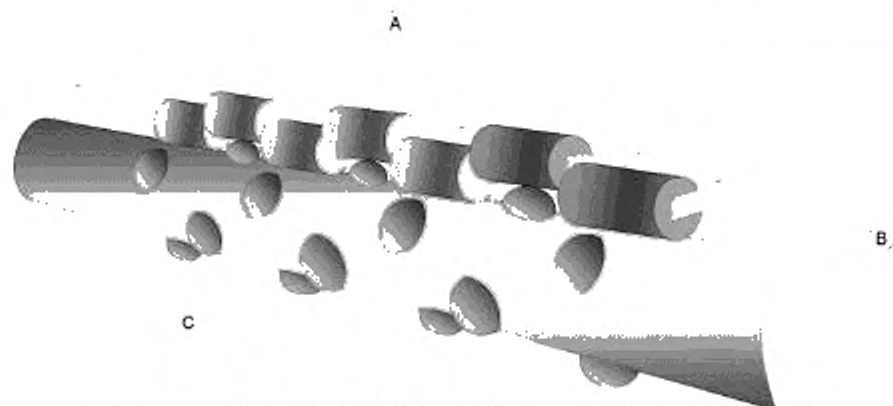
Рисунок ВВ.2 – Детальный эскиз барабана и цилиндров
