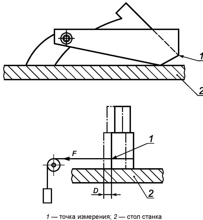
Рисунок F.3 — Испытание на устойчивость ограждения дисковой пилы, установленного на расклинивающем ноже
