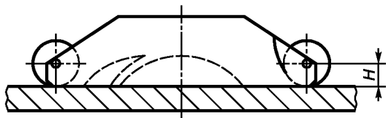
Рисунок 27 — Размеры ролика на переднем крае ограждения пильного диска, установленного на столе отдельно от расклинивающего ножа
