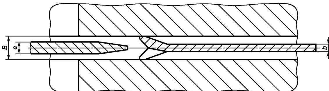
e — толщина расклинивающего ножа; b — толщина диска пилы; B — ширина пропила
