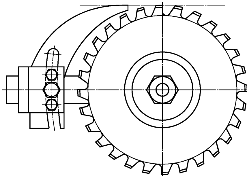
Рисунок 12 — Установка расклинивающего ножа по высоте
