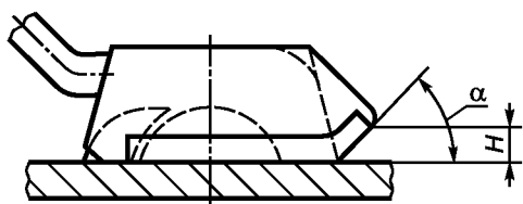
Рисунок 26 — Размеры подводящего скоса на передней части ограждения пильного диска, установленного на столе отдельно от расклинивающего ножа
