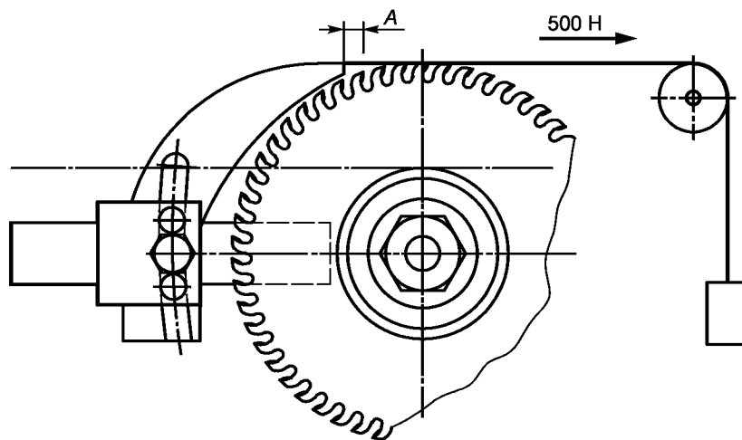
Рисунок С.1 — Испытание на продольную устойчивость расклинивающего ножа
