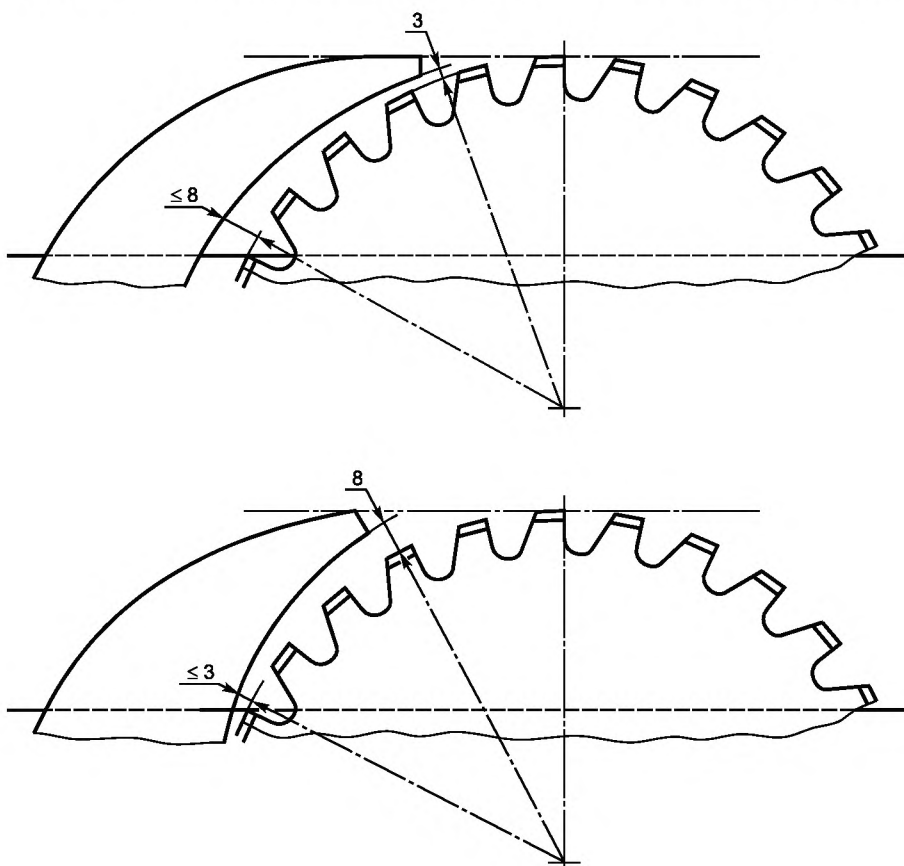
Рисунок 13 — Пределы зазоров между раскливающим ножом и дисковой пилой
