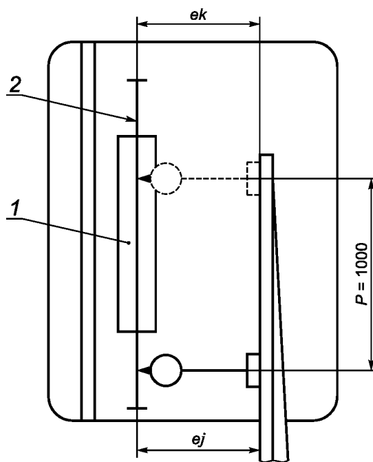
1 — дисковая пила; 2 — направляющая линейка
