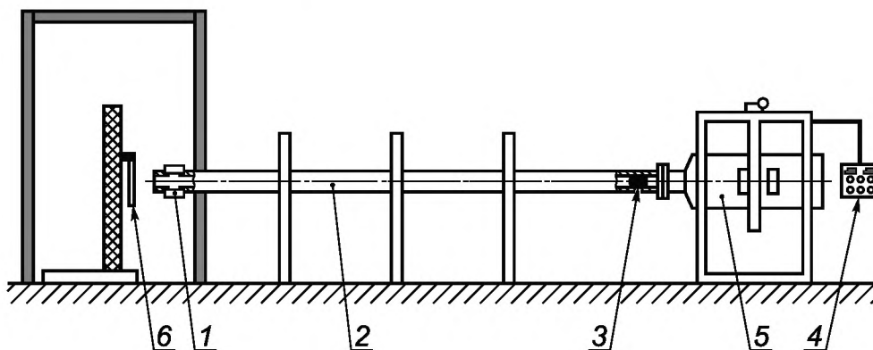
1 — измеритель скорости; 2 — ствол; 3 — перемещаемый «снаряд»; 4 — пульт управления; 5 — баллон сжатого воздуха; 6 — образец для испытания
