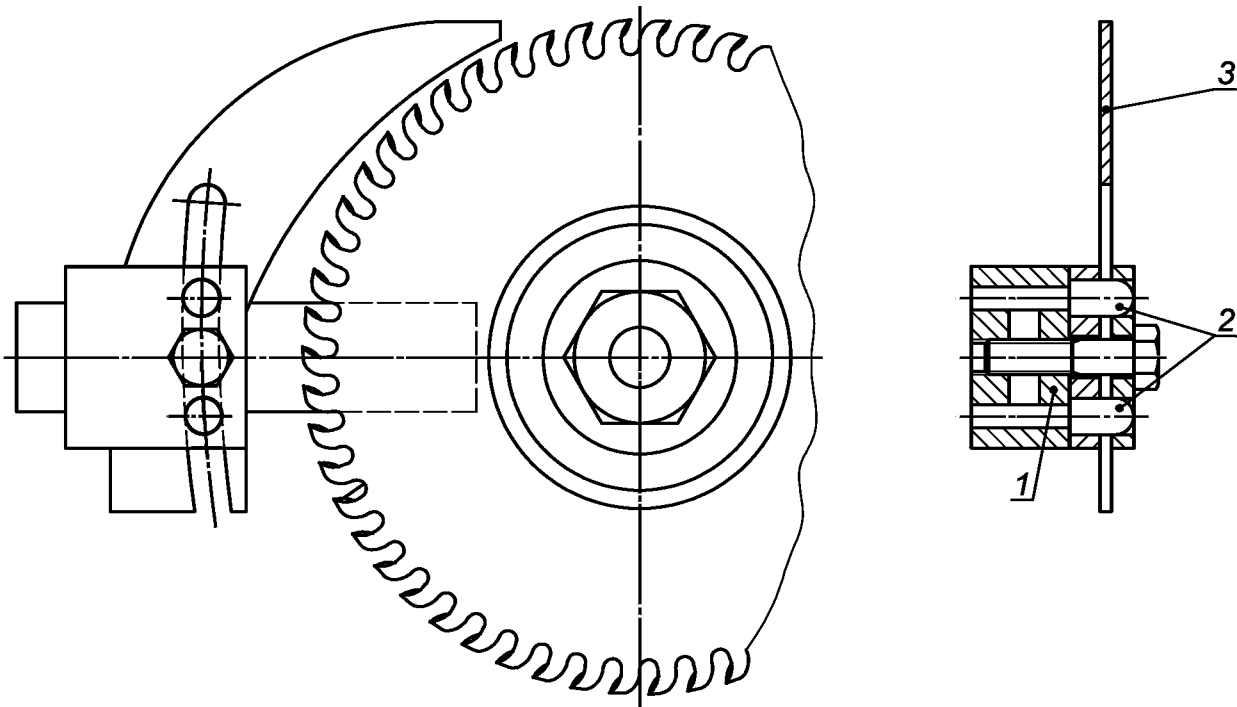
1 — держатель расклинивающего ножа; 2 — направляющие штифты; 3 — расклинивающий нож
