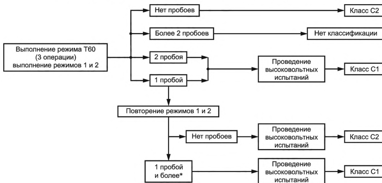
Рисунок К.1 — Процедура перекалфикации в режимах коммутации тока ненагруженных линий и кабелей
