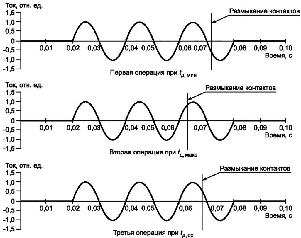
Рисунок 13 — Регулирование момента размыкания контактов относительно фазы тока при однополюсном отключении симметричного тока в режимах Т10, Т30, Т60, Т100S, Тcr1, Тcr2, Тcr3, ОР2, L90, L75, L60 выключателями с U_{ном} \geq 110 кВ
