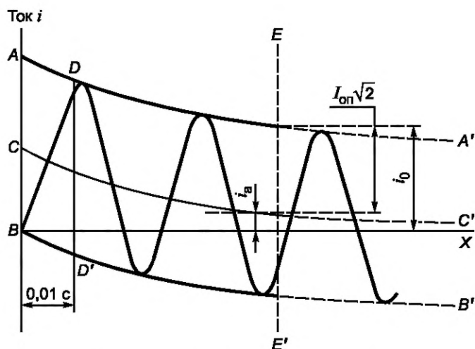
AA' и BB' — огибающие кривой тока; BX — нулевая линия; CC' — кривая смещения нулевой линии кривой тока (кривая аperiodической составляющей); DD' — момент измерения начального действующего значения периодической составляющей тока включения, EE' — момент прекращения соприкосновения дугогасительных контактов (возникновение дуги); I_{on} — действующее значение периодической составляющей тока отключения, отнесенное к моменту EE' ; i_a — аperiodическая составляющая тока отключения в момент EE' ; i_0 — амплитуда тока отключения в момент EE'
