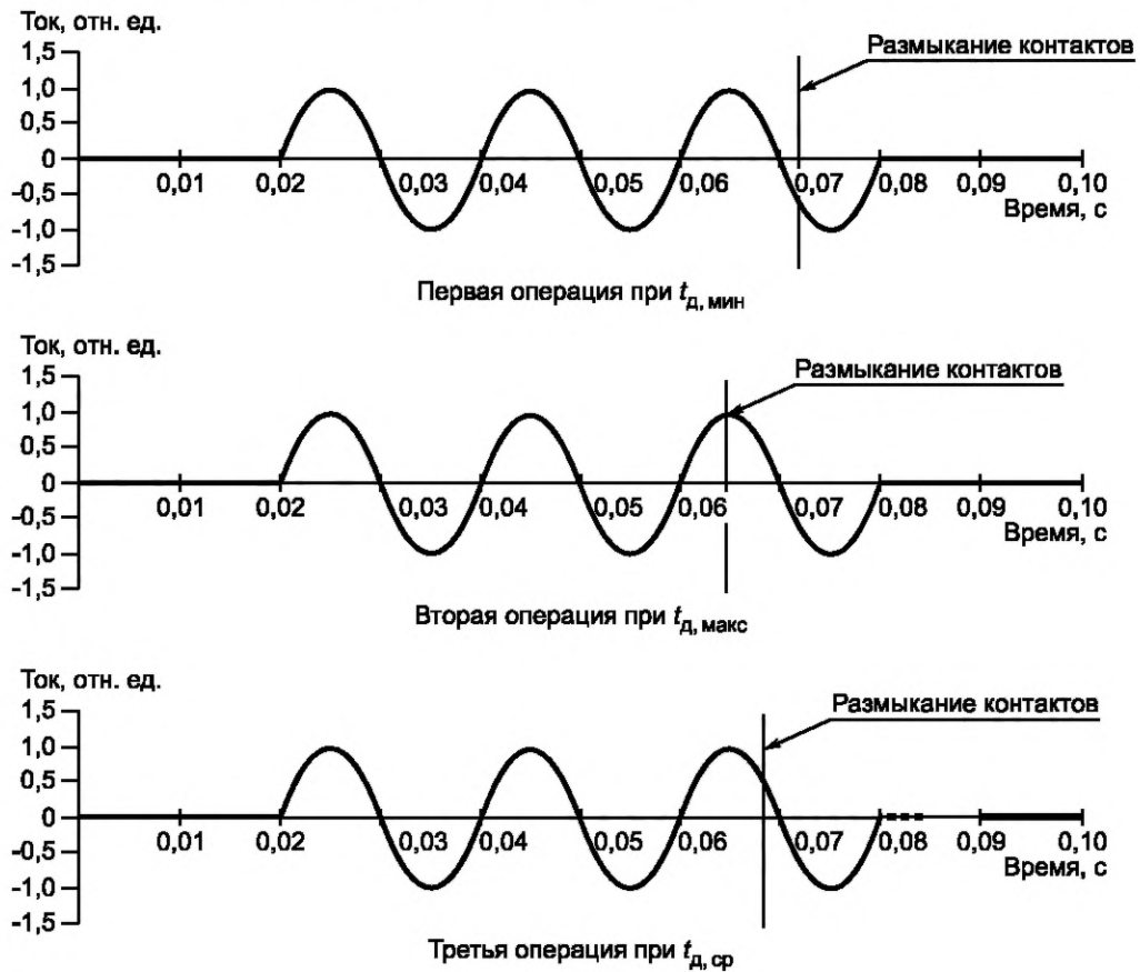
Рисунок 11 — Регулирование момента размыкания контактов относительно фазы тока при однополюсном отключении симметричного тока в режимах Т10, Т30, Т60, Т100с, Тсr1, Тсr2, Тсr3 выключателями с U_{\text{ном}} \leq 35 кВ
