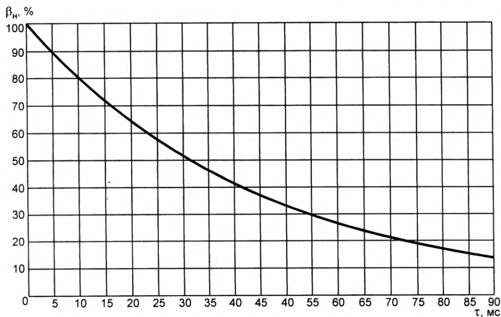
Рисунок 3 — Содержание аperiodической составляющей в процентах
