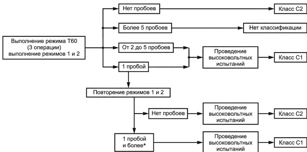
Рисунок К.2 — Процедура перекалфикации в режимах коммутации тока конденсаторных батарей
