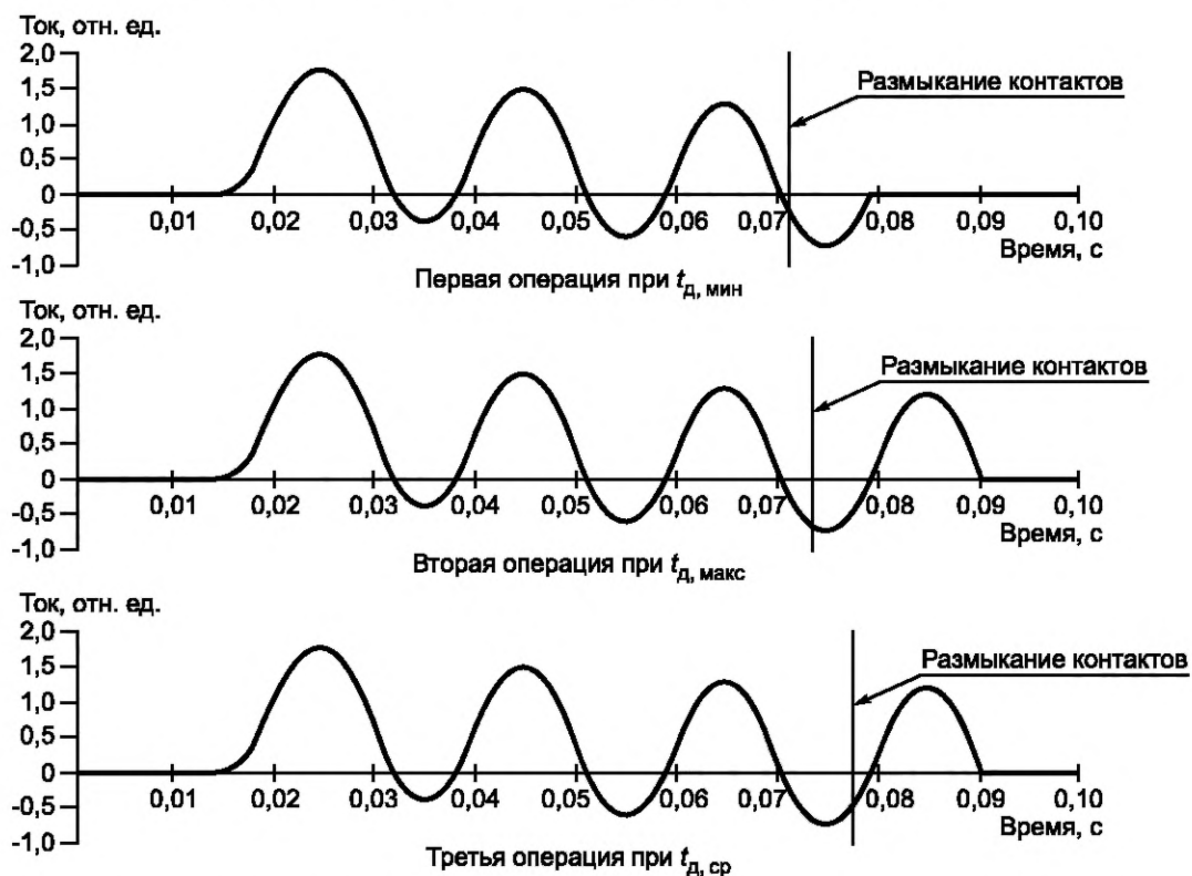
Рисунок 12 — Регулирование моментов инициирования тока и размыкания контактов при однополюсном отключении тока в режиме Т100а выключателями с U_{ном} \leq 35 кВ
