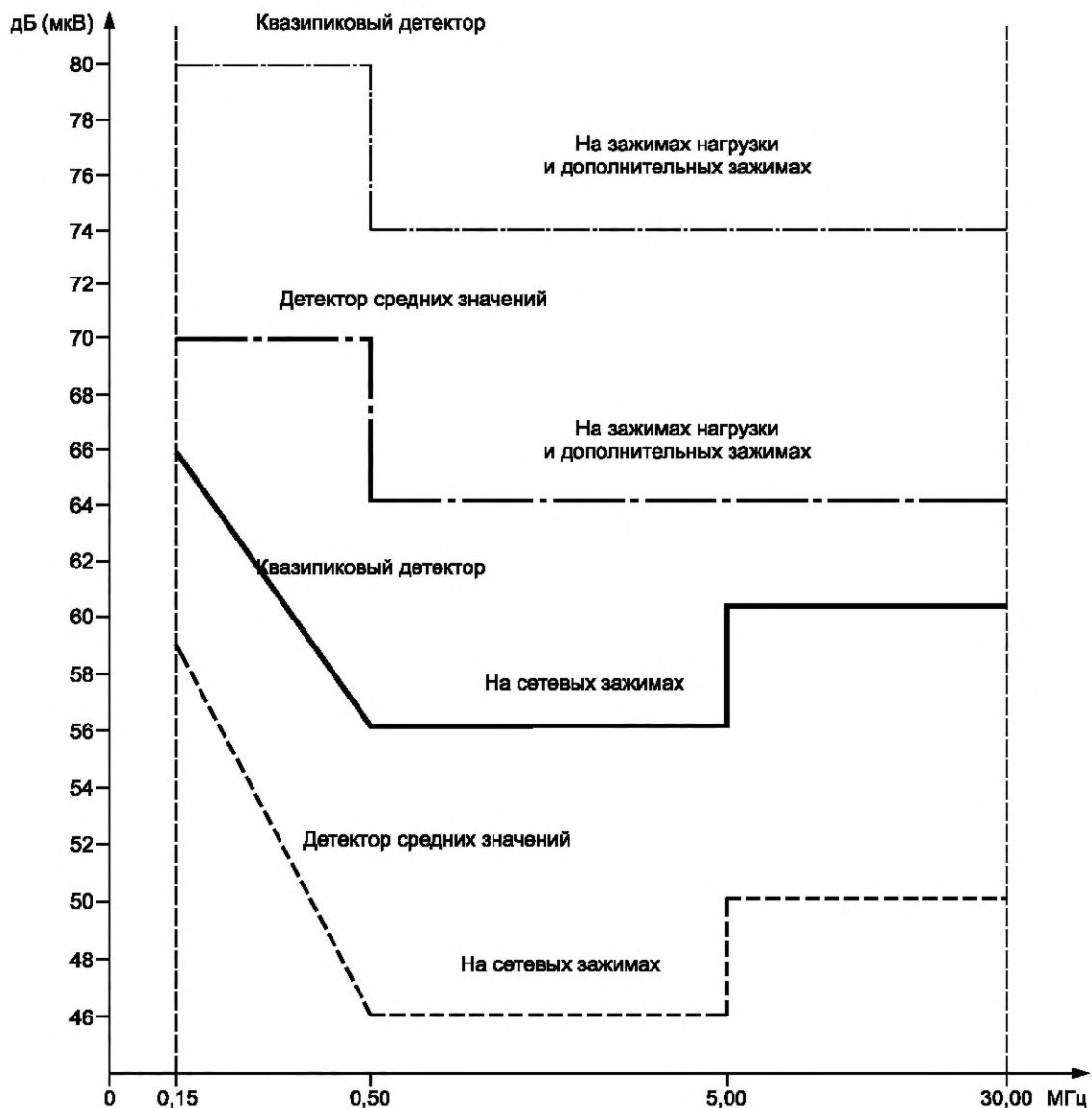
Рисунок 2 — Графическое представление норм, регулирующие устройства (см. 4.1.1)
