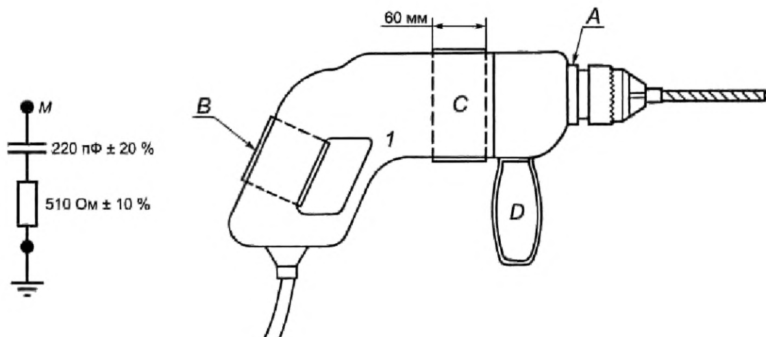
Рисунок 8а) — Элемент RC
