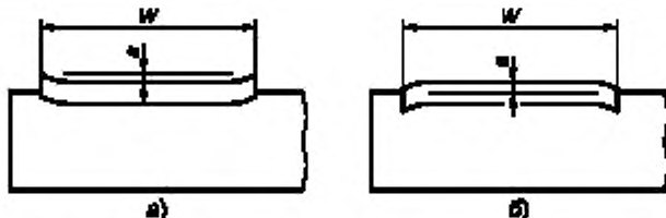
Рисунок 3 — Профиль поверхности
