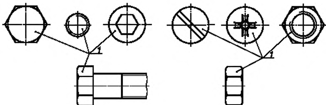
1 — поверхности измерения
