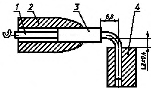
1 — вывод ЭРИ; 2 — зажим; 3 — корпус изделия; 4 — держатель
