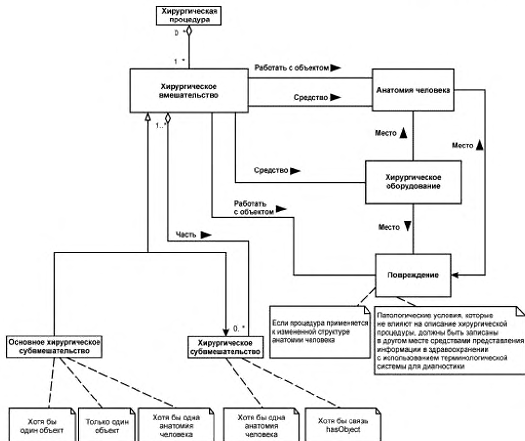
Рисунок 1 — UML диаграмма
