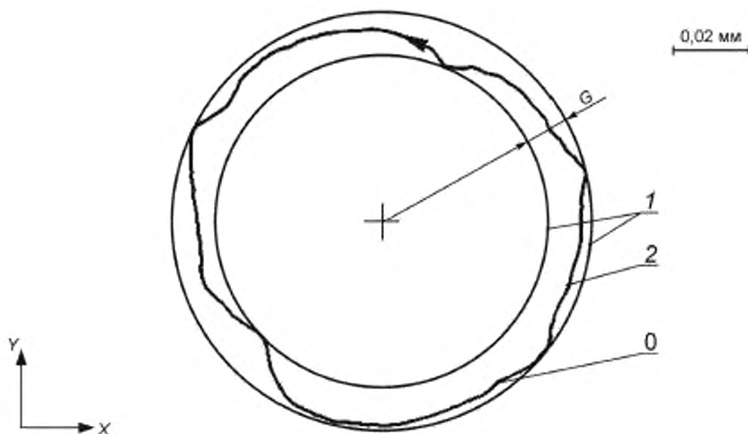
Рисунок 2 — Измерение кругового отклонения G
