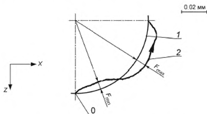
Рисунок 3 — Измерение радиального отклонения F
