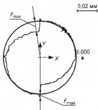
Рисунок 6 — Пример представления данных для радиального отклонения F
