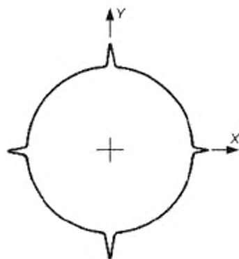
Рисунок В.5 — Пиковые отклонения с интервалом 90° вследствие реверсирования
