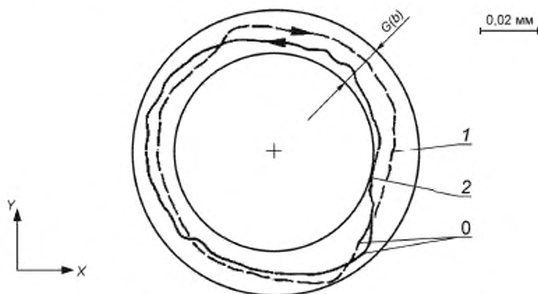
Рисунок 1 — Измерение двунаправленного отклонения
