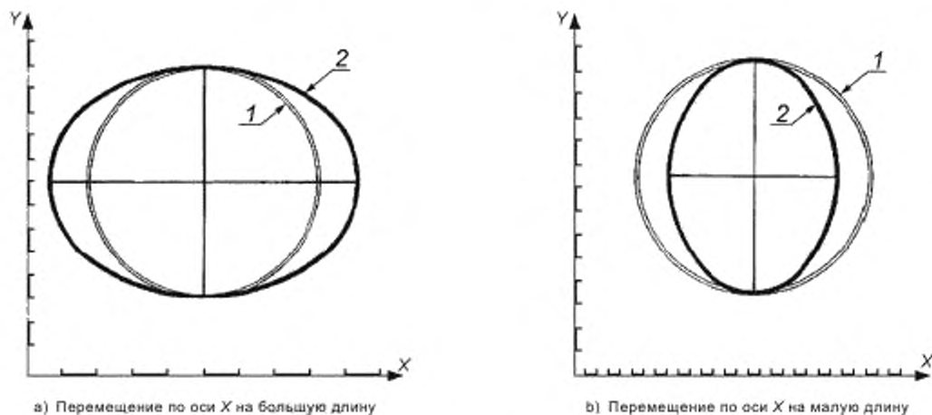
Рисунок В.1 — Влияние на круговые траектории перемещений на большую и малую длины по оси
