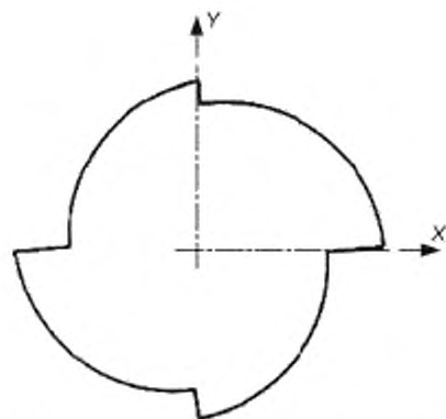
Рисунок В.4 — Переходы с интервалом 90° вследствие реверсирования
