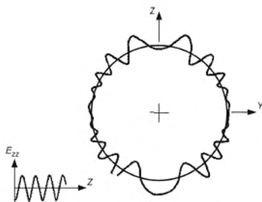
Рисунок В.3 — Влияние циклических отклонений Z
