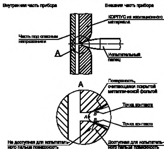
Рисунок 2 — Пример оценки УСИЛЕННОЙ ИЗОЛЯЦИИ
