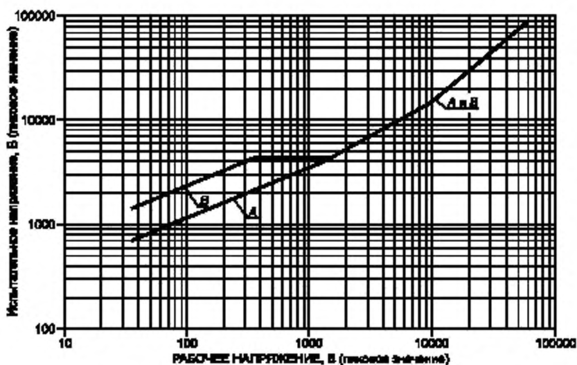
Рисунок 7 — Испытательное напряжение
