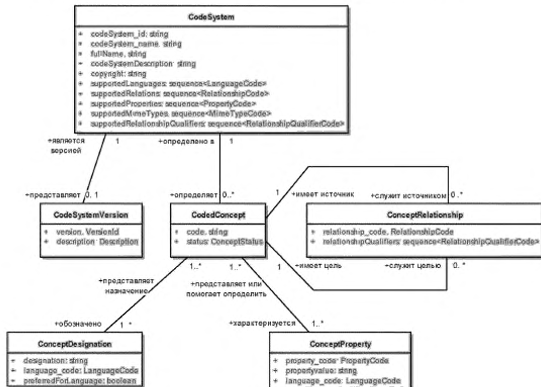
Рисунок 6 — Классы, образующие систему кодирования
