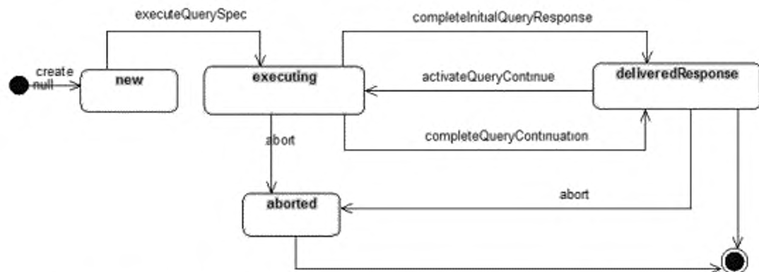
Рисунок А.14 — Диаграмма перехода состояний класса QueryEvent (событие запроса)
