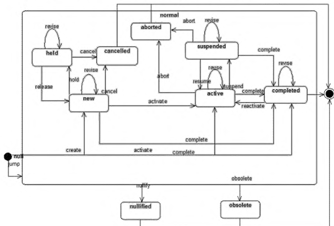
Рисунок A.5 — Диаграмма перехода состояний класса Act (действие)
