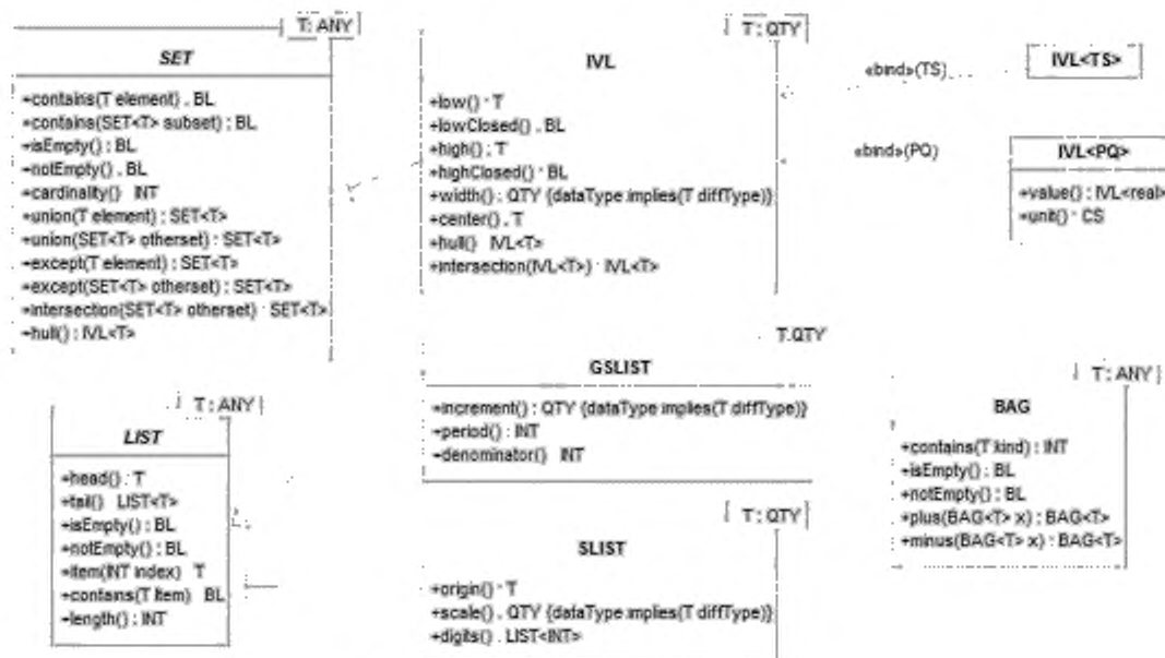
Рисунок В.11 — Типы данных общих коллекций
