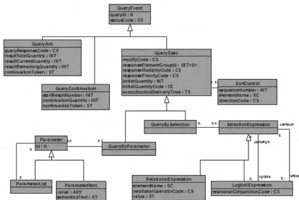
Рисунок A.12 — Диаграмма классов предметной области QueryControl (управление запросами)
