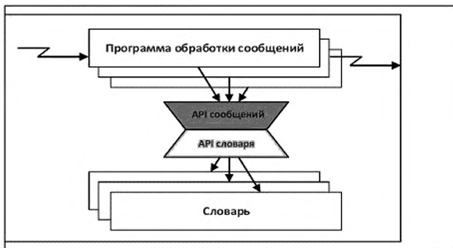
Рисунок 1 — API сообщений и словаря
