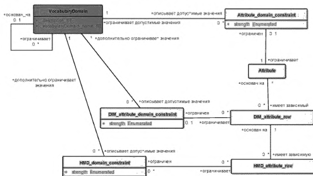
Рисунок 3 — Атрибуты модели RIM и словарные домены
