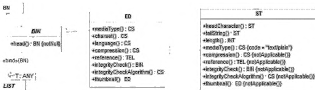
Рисунок В.3 — Обзор мультимедийных и текстовых типов данных
