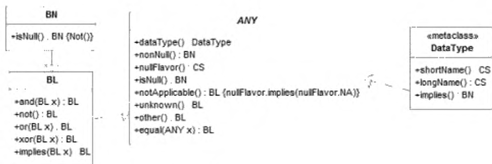
Рисунок В.2 — Фундаментальные типы данных
