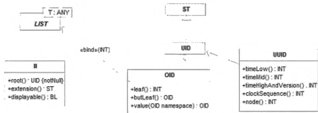
Рисунок B.5 — Типы данных экземпляров идентификаторов
