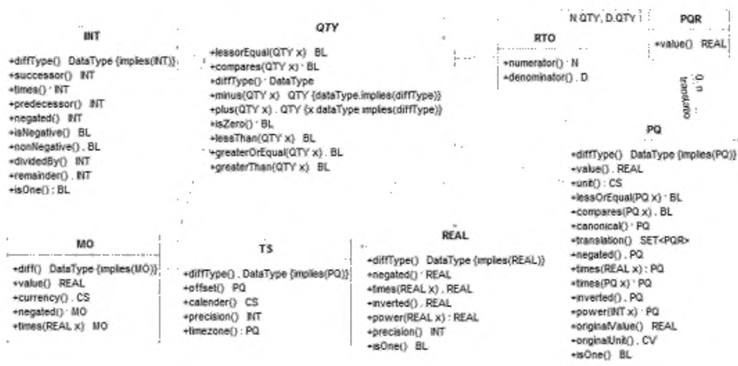
Рисунок В.9 — Типы данных количества
