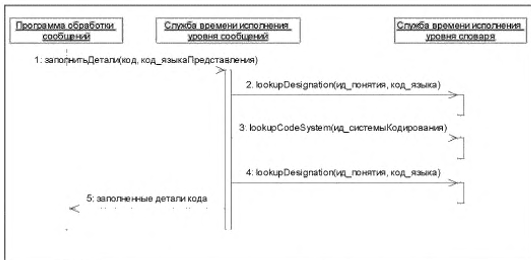
Рисунок 2 — Пример взаимодействия с API сообщений и словаря
