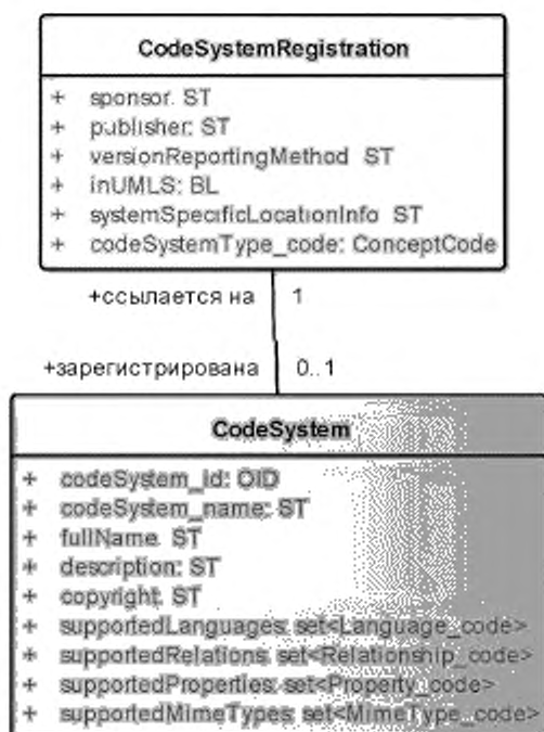
Рисунок 5 — Зарегистрированная система кодирования
