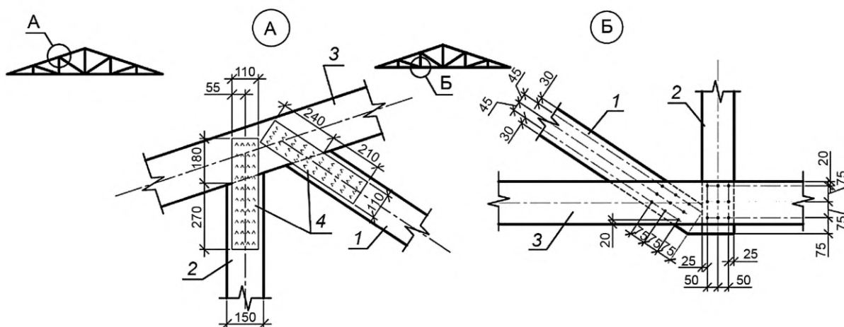
а — узловое соединение на металлических зубчатых пластинах (МЗП); б — узловое соединение на гвоздях
