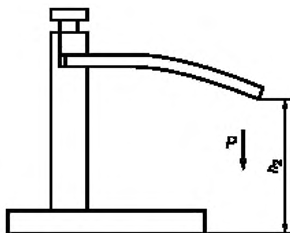
Рисунок 8 — Карта в зажимном устройстве во время нагрузки
