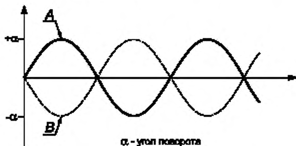
Рисунок 13 — Циклы скручивания
