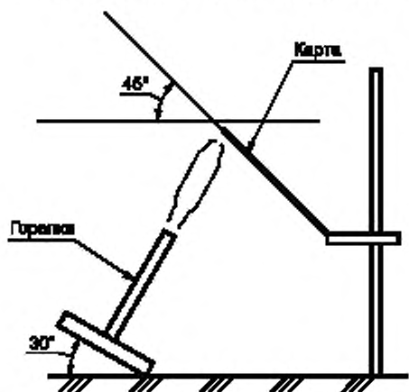
Рисунок 14 — Расположение карты и горелки
