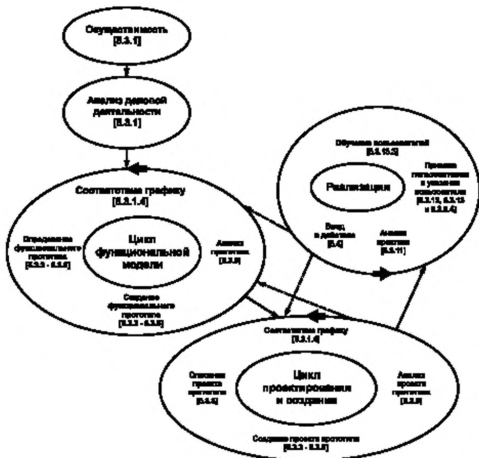
Рисунок D.3 — Пример ускоренной разработки приложения (УРП)
