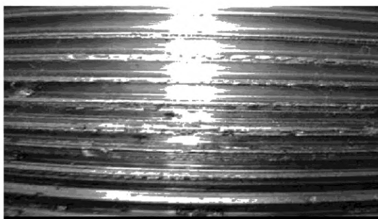
в) Задиры на наружной резьбе после свинчивания
