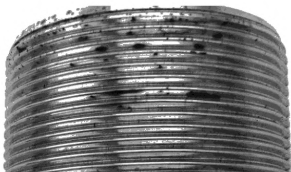
б) Следы коррозии на наружной резьбе
