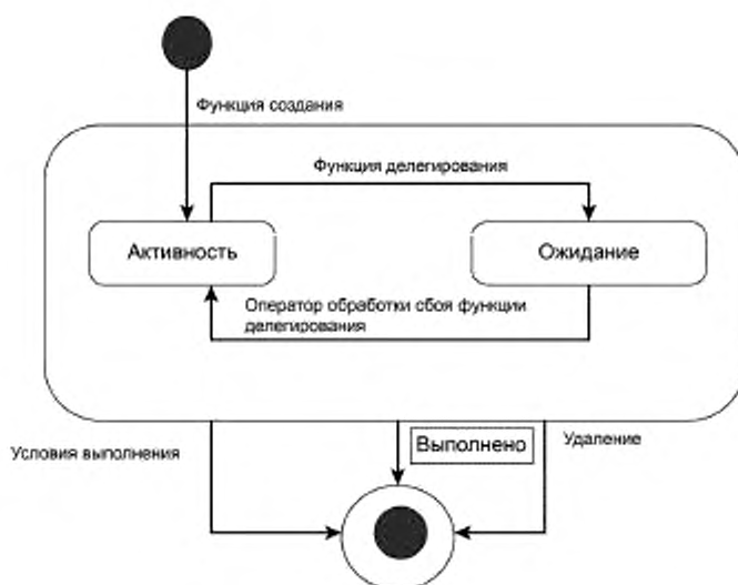
Рисунок А.6 — Нормативный маркер жизненного цикла
