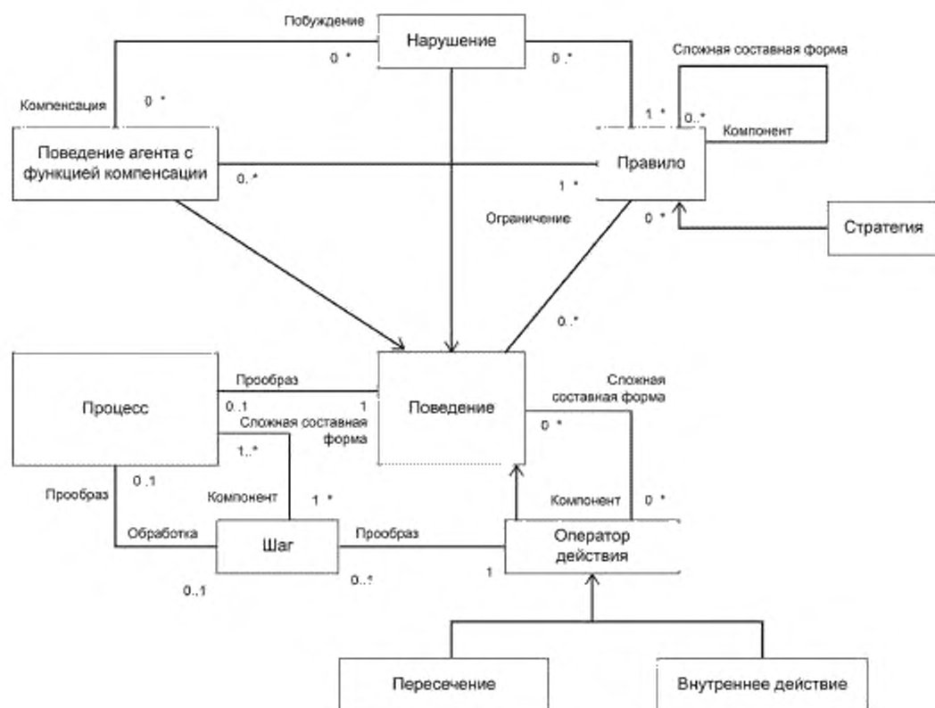
Рисунок А.3 — Концепции поведения
