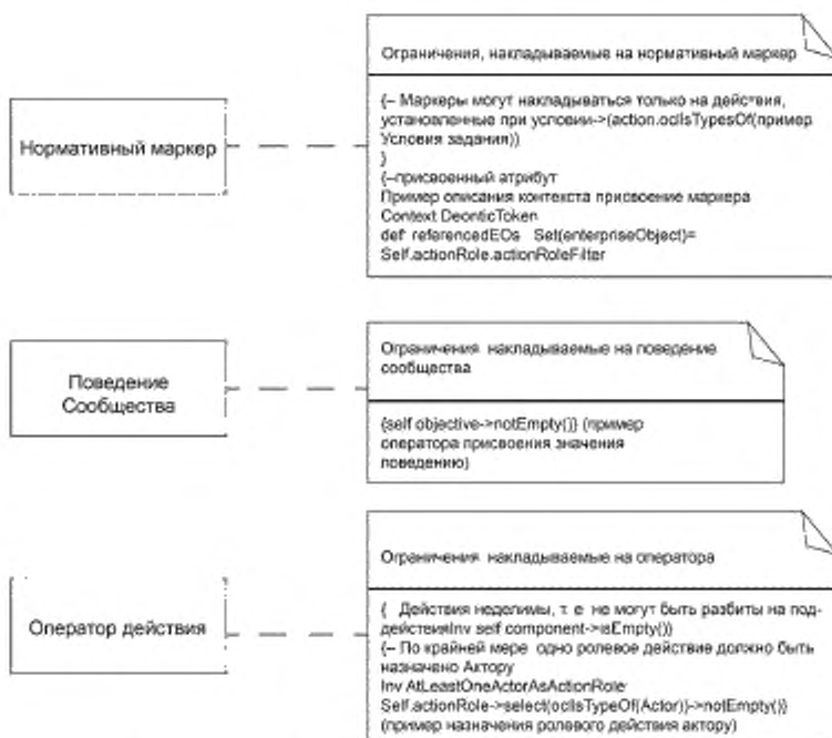
Рисунок А.2 — Понятия (концепты) описания сообщения
