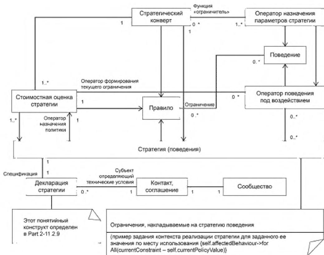
Рисунок А.4 — Понятия описания стратегий поведения
