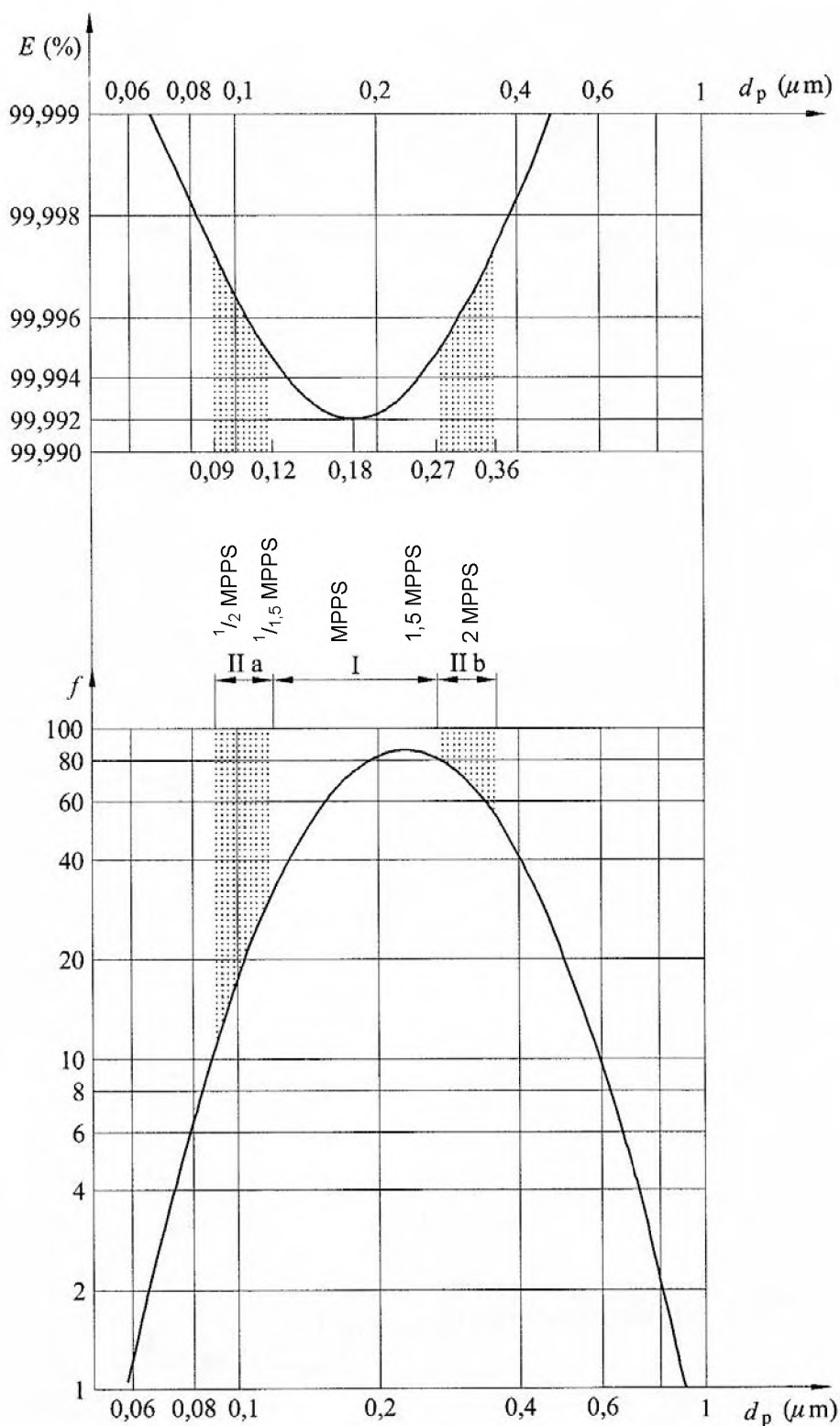
Р и с у н о к 4 — Фракциональная эффективность E и допустимые пределы чувствительности относительно минимальной эффективности (MPPS = 0,18 мкм) и численное распределение f полидисперсного контрольного аэрозоля с диаметром частиц d_p = 0,23 мкм
