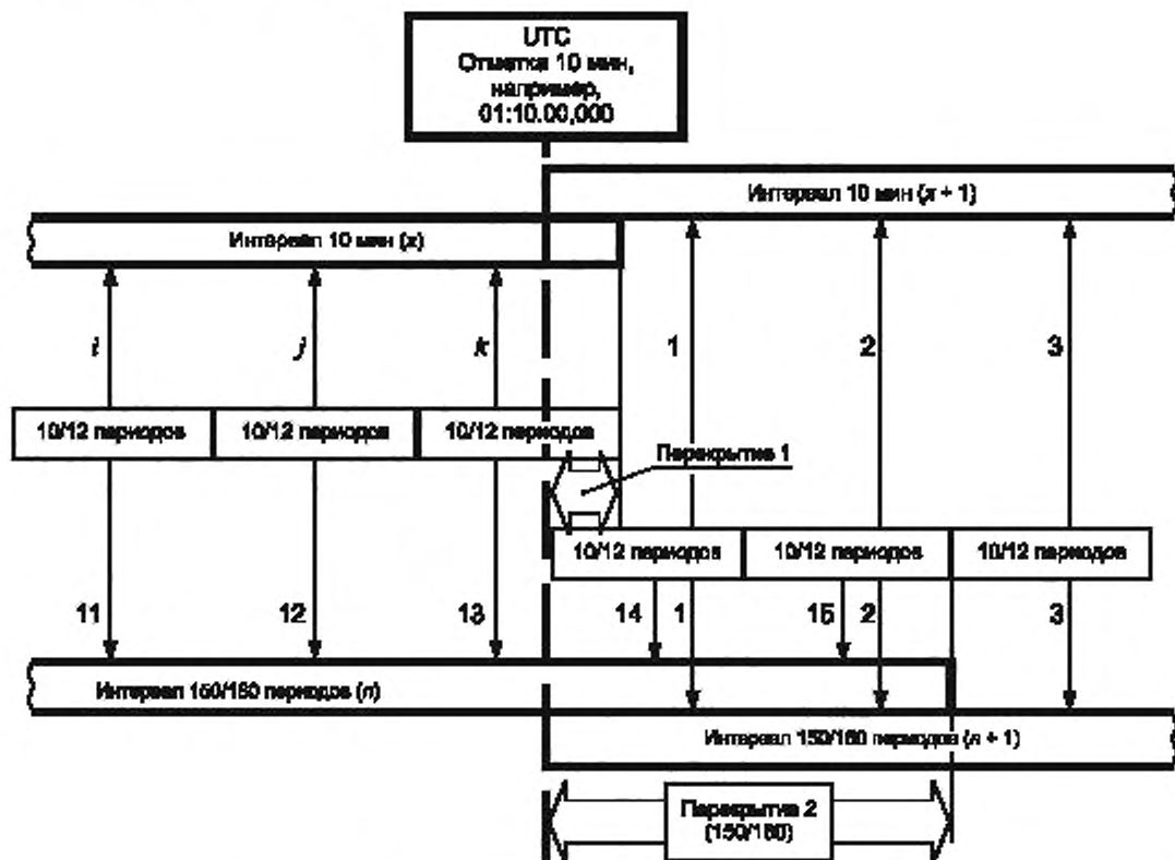
Рисунок 2 — Синхронизация объединенных интервалов для класса А
