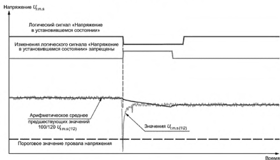
Рисунок 7 — Событие, не относящееся к быстрому изменению напряжения.
