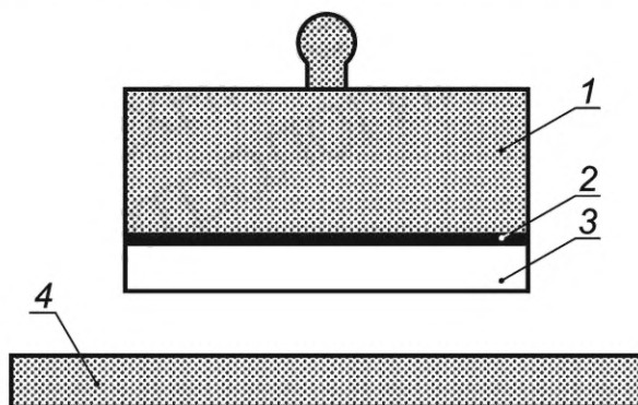
АТ-1 – адгезионный отрыв на границе «образец–бетонная плита»
